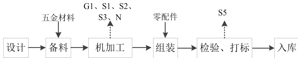
图 2-2 工装治具生产工艺流程图
