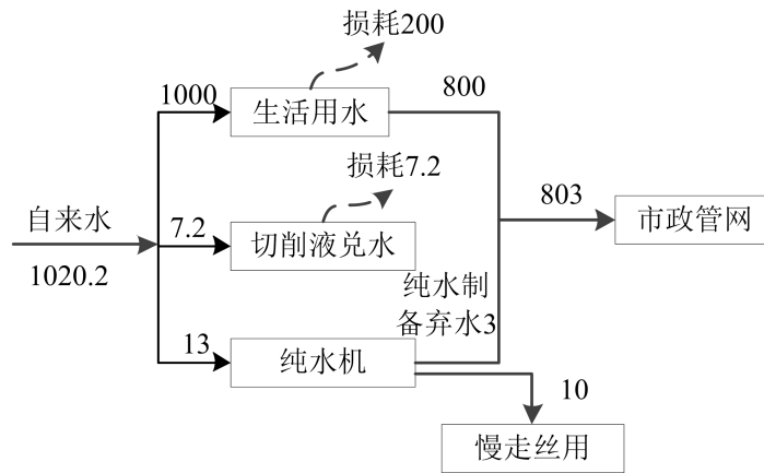
图 2-3 现有项目水平衡图
