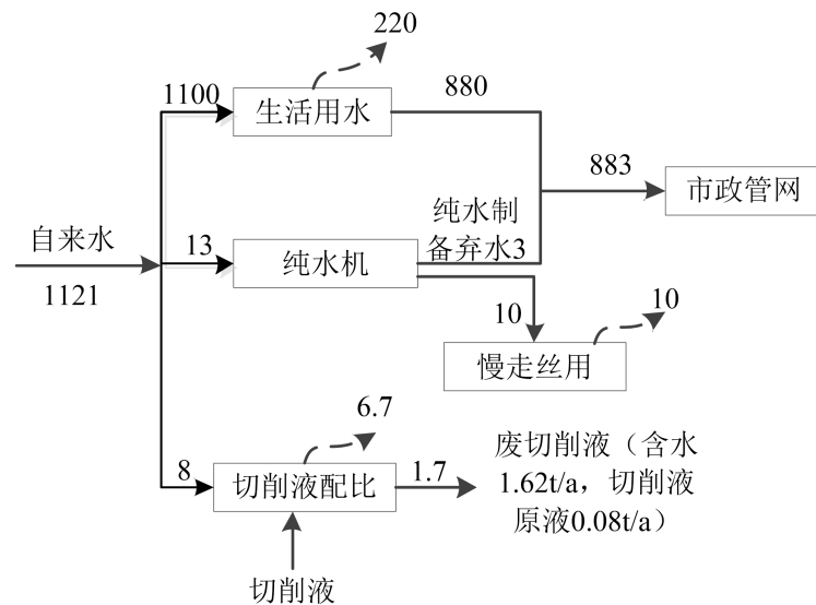
图 4-3 本项目水平衡图 (t/a)
