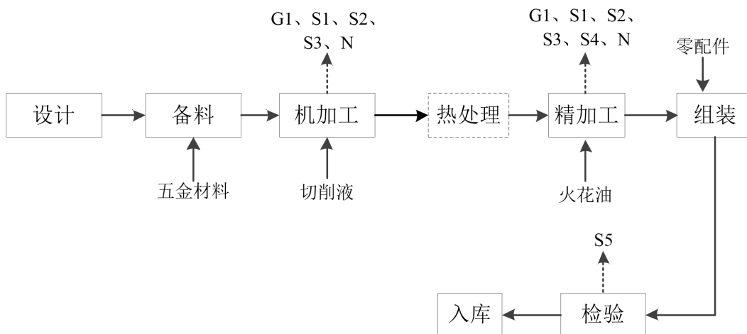
图2-1 模具生产工艺流程图
