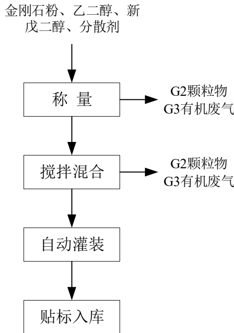
图 2-3 研磨液生产工艺流程图
