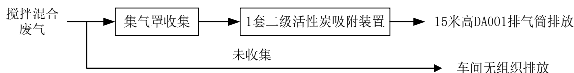
图 4-1 本项目废气收集、处理情况
