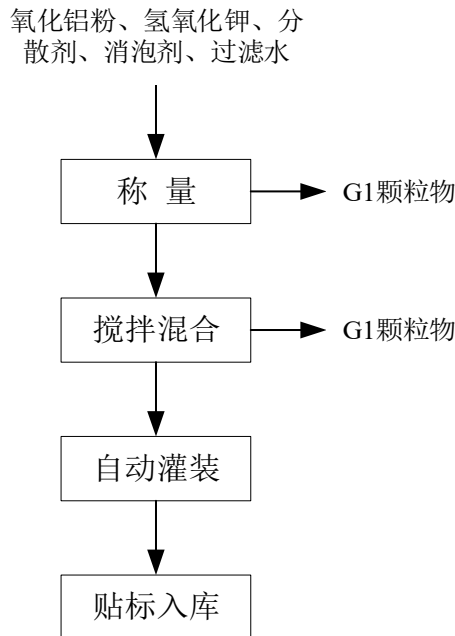
图 2-2 抛光液生产工艺流程图
