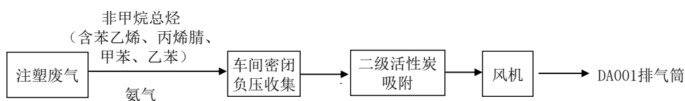
图 4-1 废气收集处理工艺流程图
