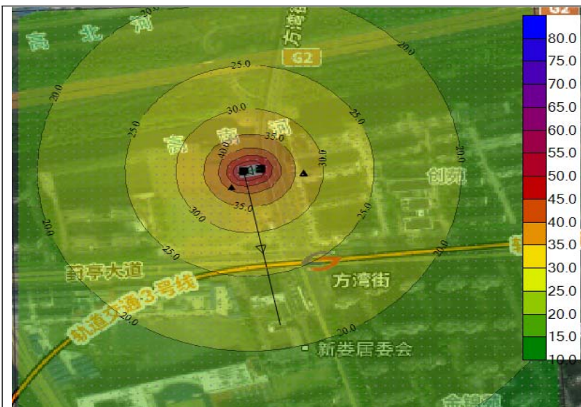
近期昼间等声级线图
