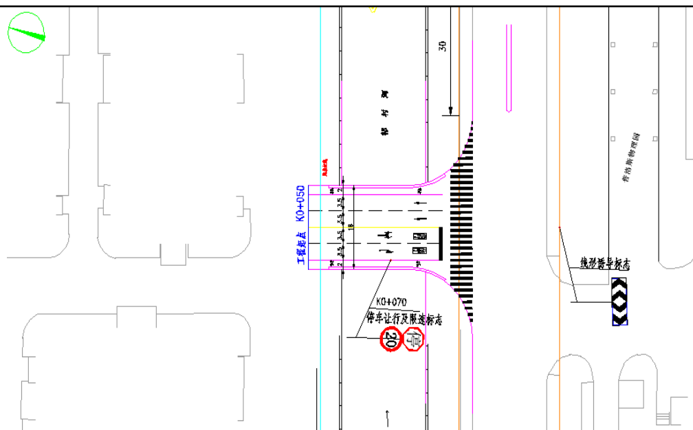
图 2-3 贸易功能区医药配送中心项目出入口桥梁项目布置图
