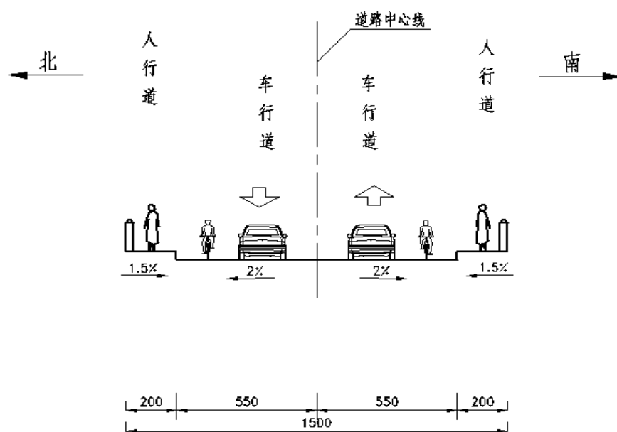
图 2-7 2.5 产业园三期三区出入口桥梁项目处横断面
