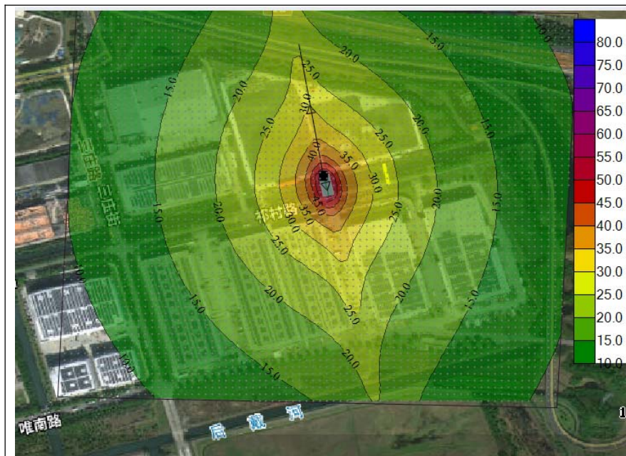
近期昼间等声级线图
