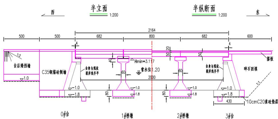
图 2-8 2.5 产业园三期三区出入口桥梁项目桥梁立面
