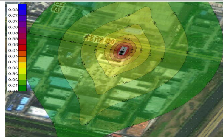
中期夜间等声级线图
