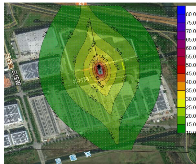
中期夜间等声级线图
