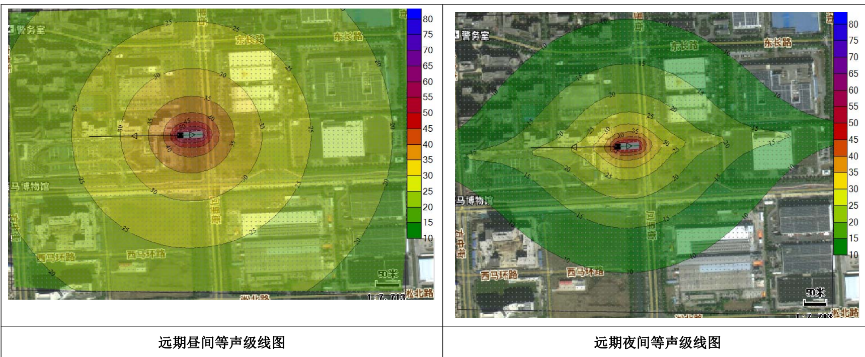
图4-82.5产业园三期三区出入口桥梁项目路段噪声水平衰减等声级线图
