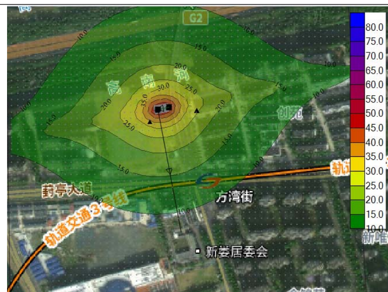
近期夜间等声级线图
