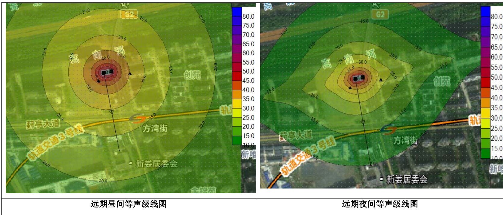
图4-6跨塘保利发展住宅项目东侧出入口噪声水平衰减等声级线图
