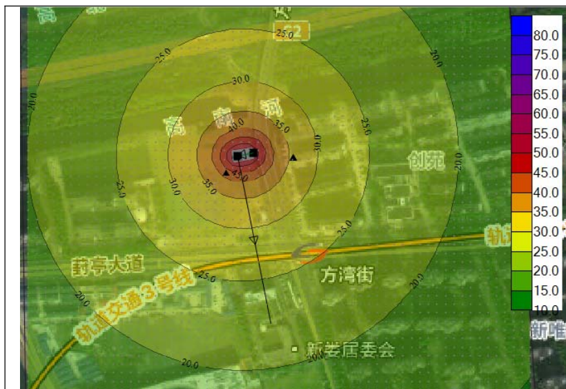
中期昼间等声级线图
