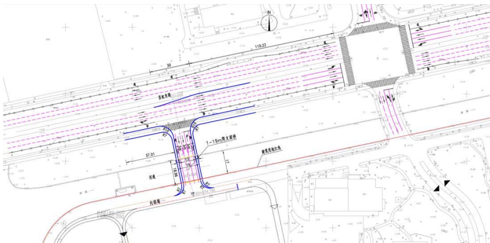
图 2-9 东沙湖基金小镇三期项目北侧桥梁工程平面布置
