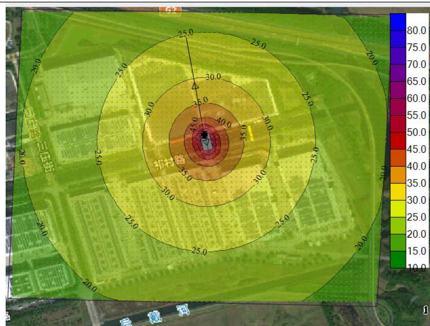
中期昼间等声级线图
