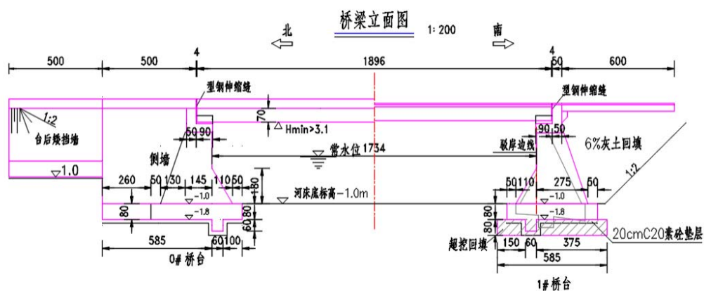
图 2-11 东沙湖基金小镇三期项目北侧桥梁工程桥梁立面图
