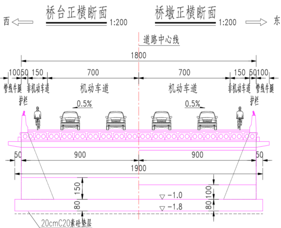
图 2-4 贸易功能区医药配送中心项目出入口横断面图
