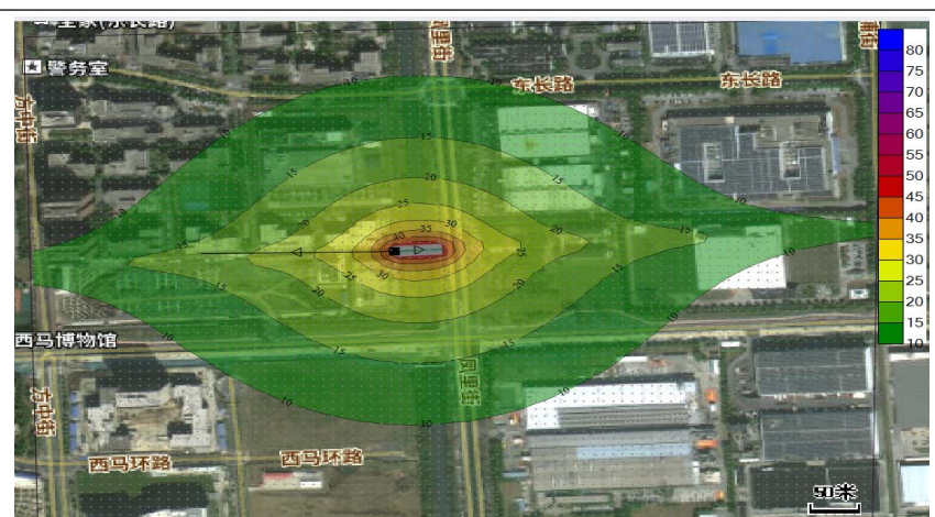
近期夜间等声级线图
