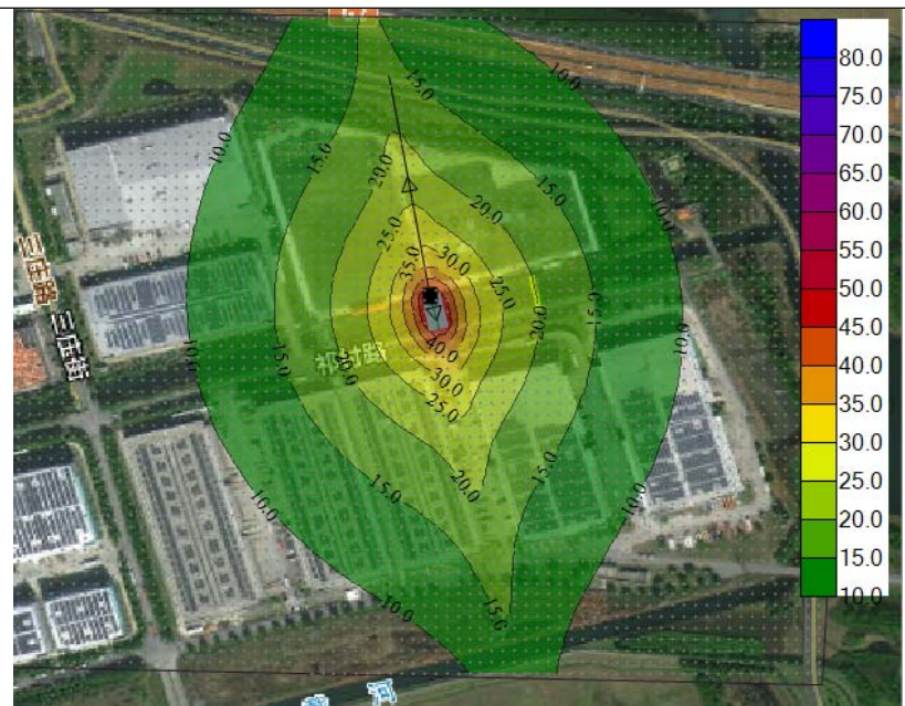
近期夜间等声级线图
