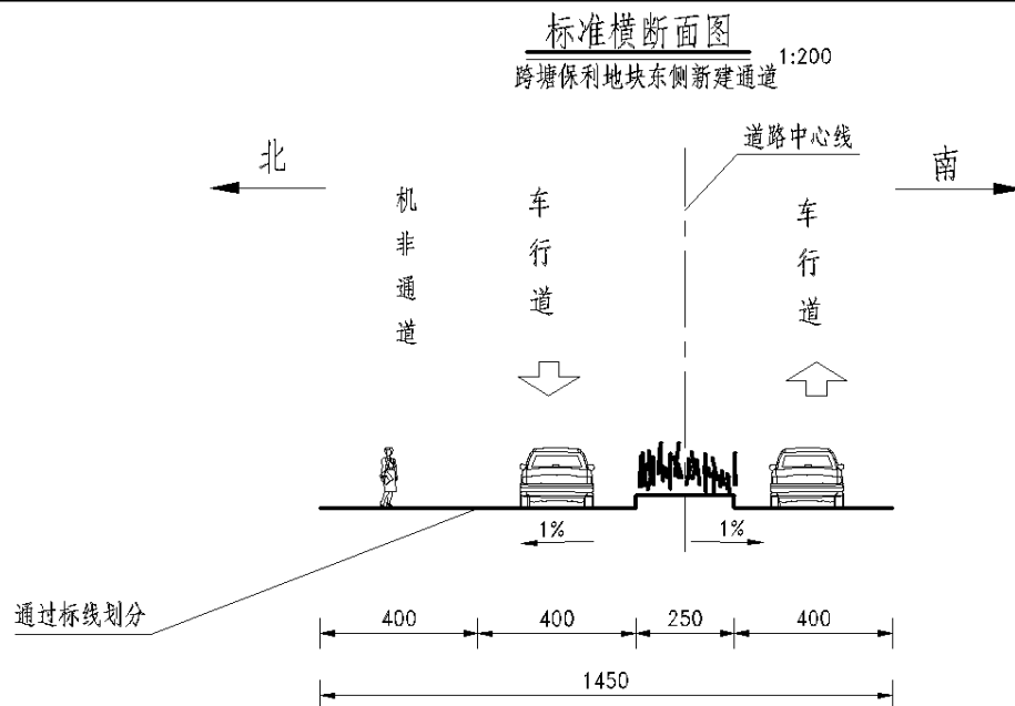
图 2-2 跨塘保利发展住宅项目东侧出入口道路典型横断面
