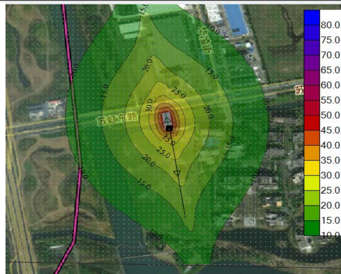
近期夜间等声级线图
