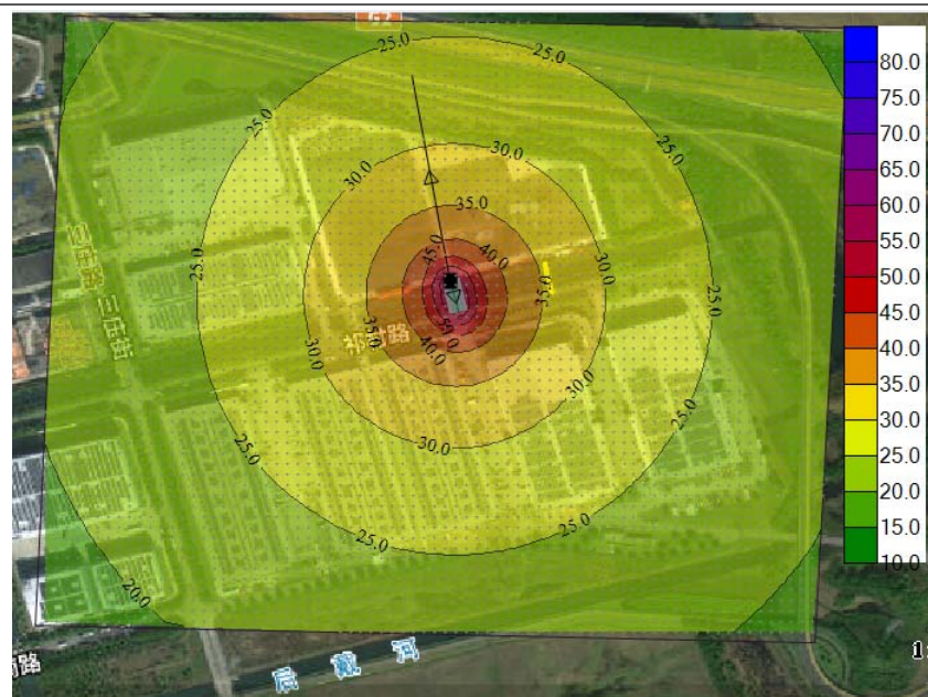
远期昼间等声级线图
