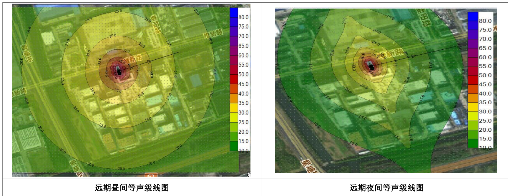
图4-10生物医药产业园六期北侧（唯新路）出入口噪声水平衰减等声级线图
