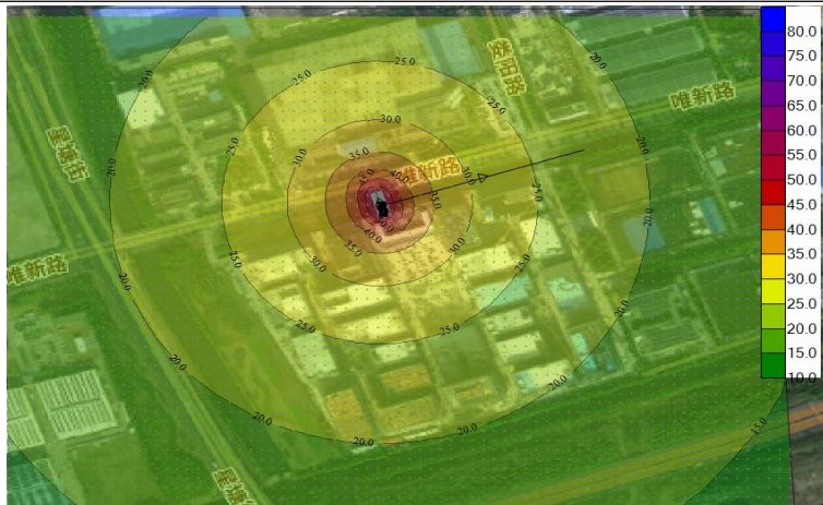
近期昼间等声级线图
