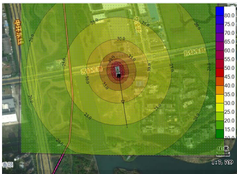
远期昼间等声级线图
