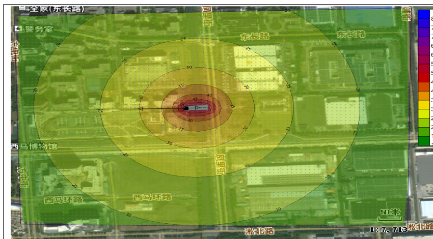
近期昼间等声级线图
