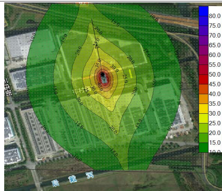
远期夜间等声级线图
