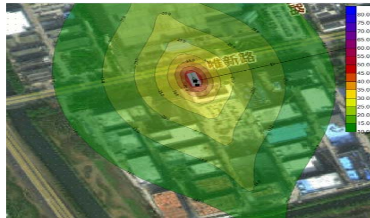
近期夜间等声级线图
