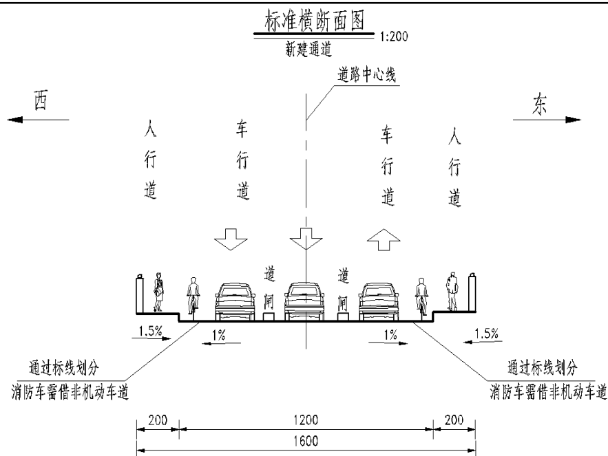
图 2-10 东沙湖基金小镇三期项目北侧桥梁工程道路典型横断面图
