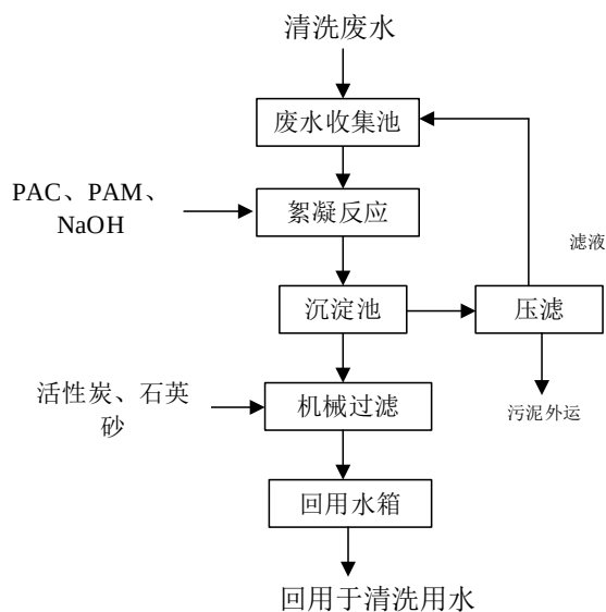
图 4-2 清洗废水处理工艺流程图
