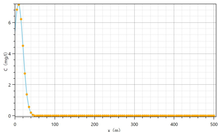
图 6.2-3 瞬时泄漏 100 天时下流 COD Mn 浓度场
