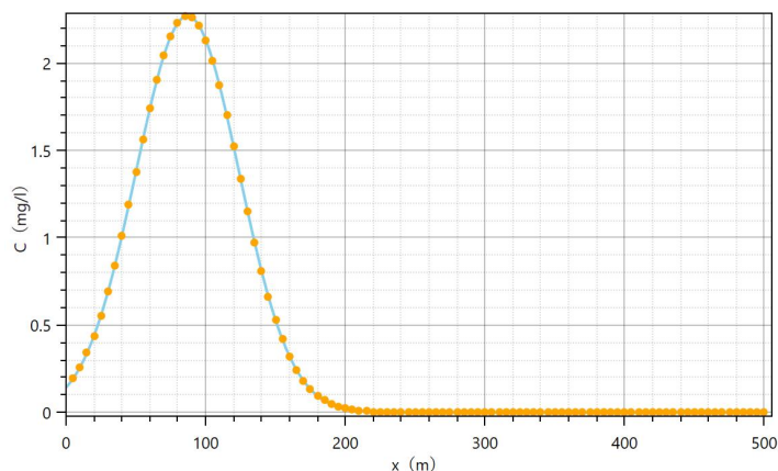
图 6.2-5 泄漏 1000 天后地下水中 COD Mn 浓度分布
