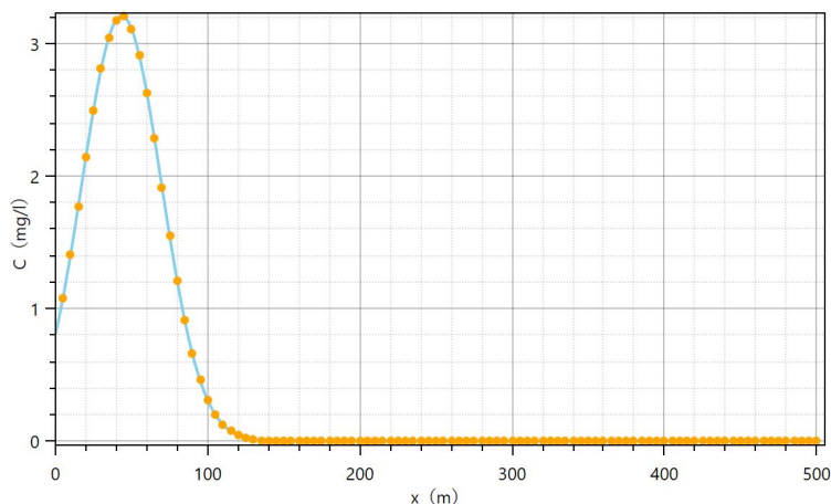
图 6.2-4 瞬时泄漏 500 天时下流 COD Mn 浓度场
