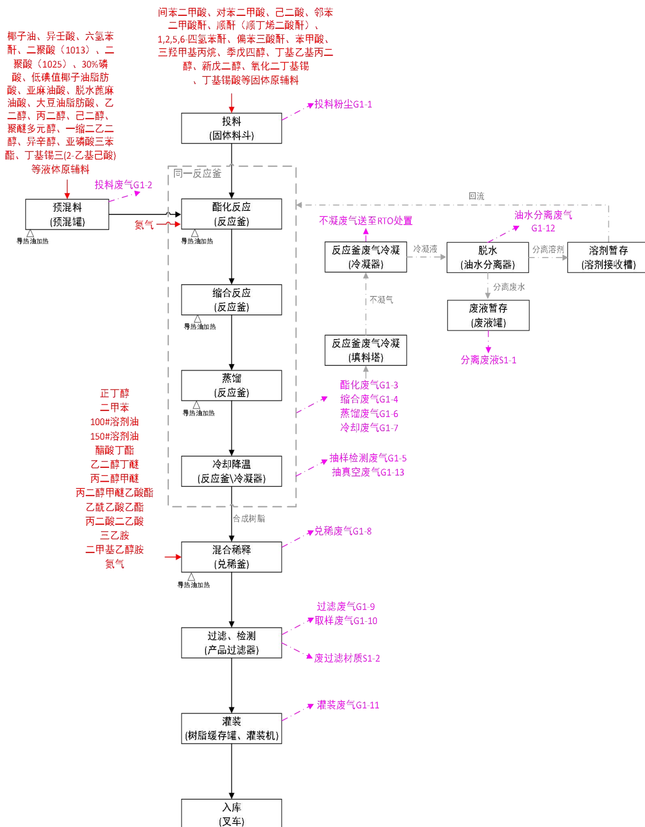
图 4.2-1 无油醇酸树脂生产工艺流程图
