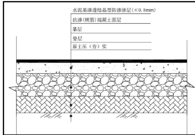
图 7.5-1 地下水重点防渗区域防渗结构图
