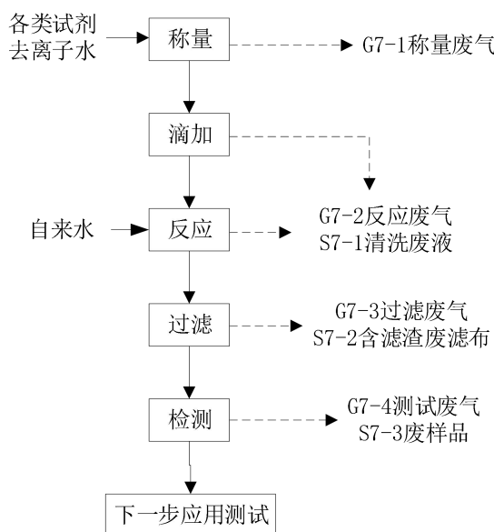
图 4.2-6 产品研发工艺流程图
