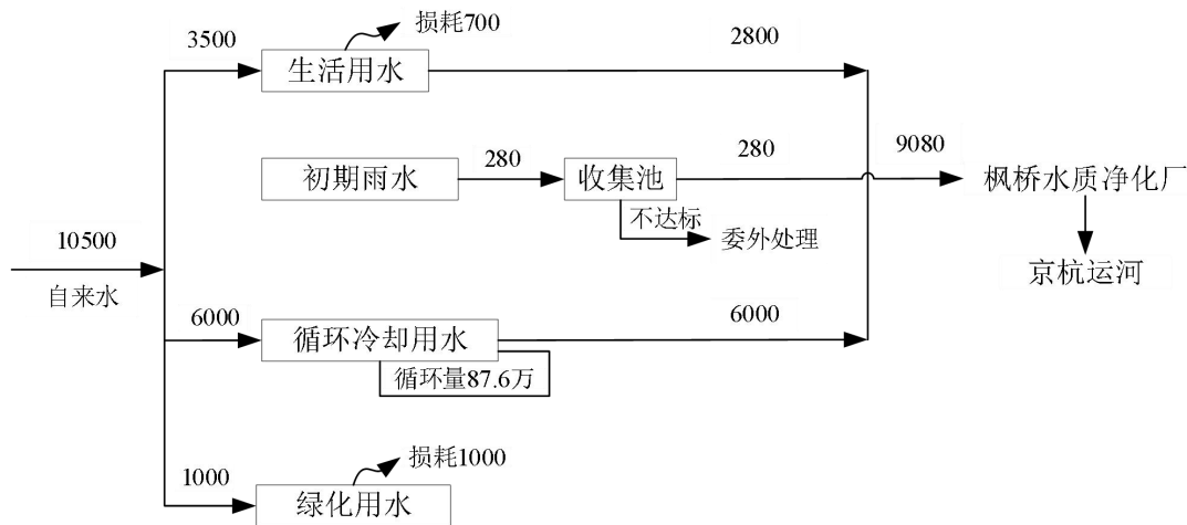
图 3.8-1 现有项目全厂水平衡图（单位：t/a）
