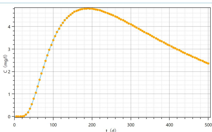
图 6.5-6 下游东侧厂界 23m 处地下水中 COD Mn 浓度随时间变化情况
