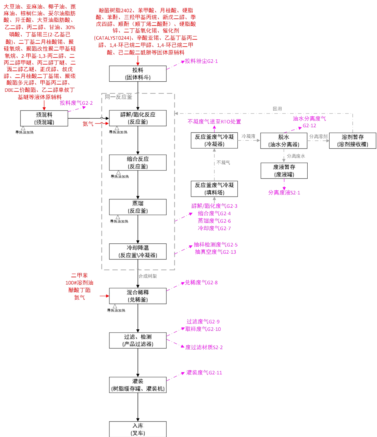
图 4.2-2 醇酸树脂生产工艺流程图
