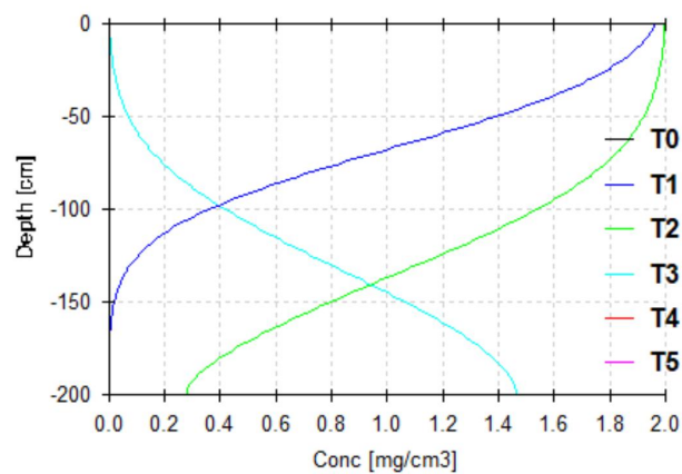
图 6.2-5 不同水平二甲苯沿土壤迁移模拟结果图
