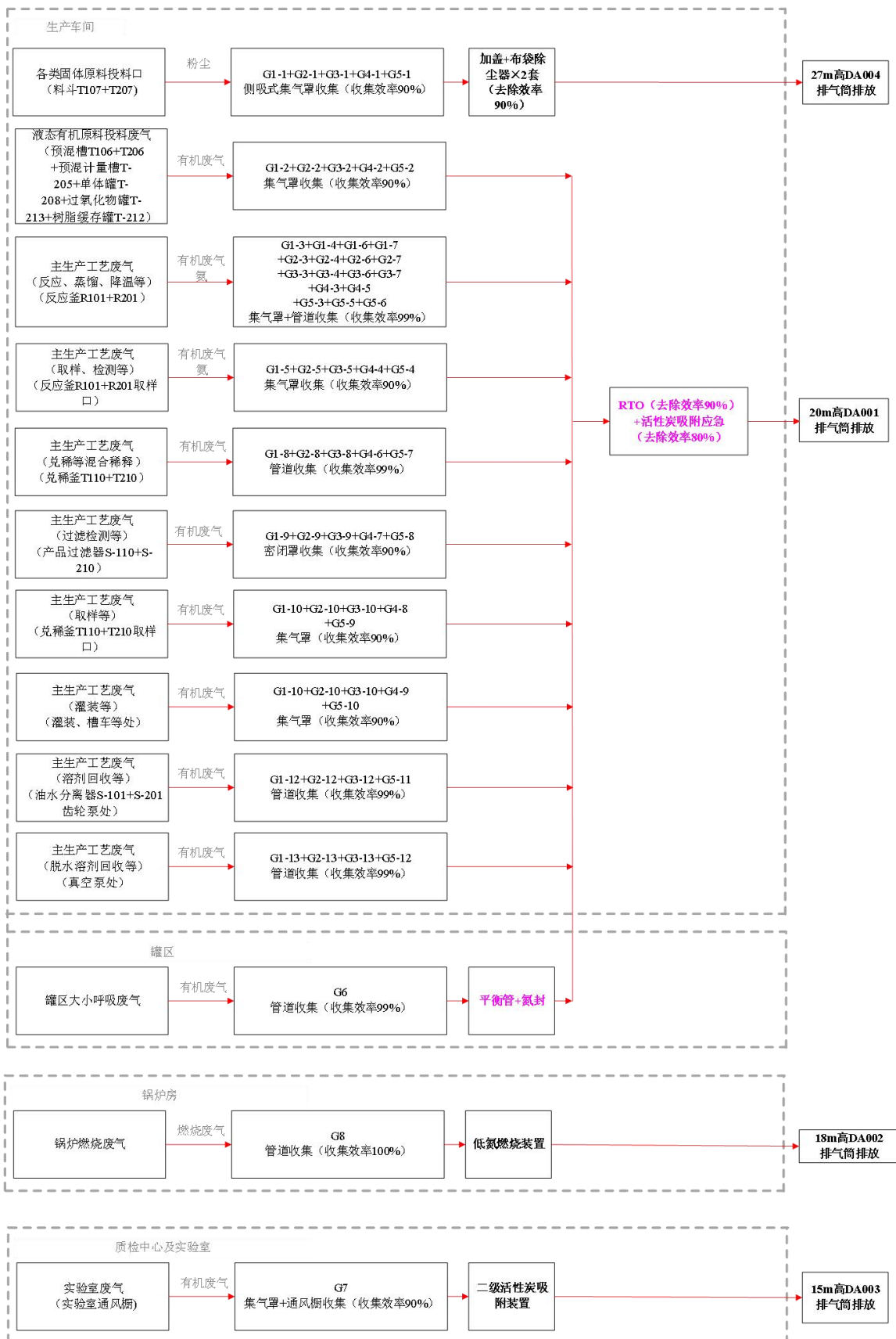
图 7.1-1 技改后全厂废气收集处理示意图
