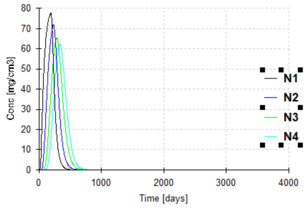
图 6.2-2 不同时间 COD 沿土壤迁移模拟结果图
