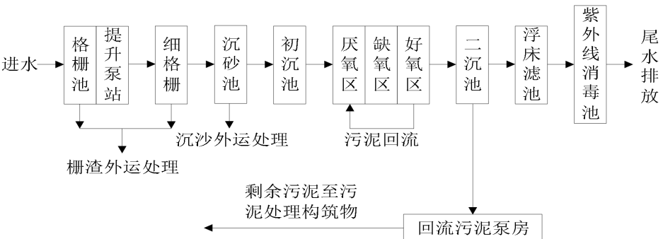
图 4-1 园区第一污水处理厂工艺流程图
