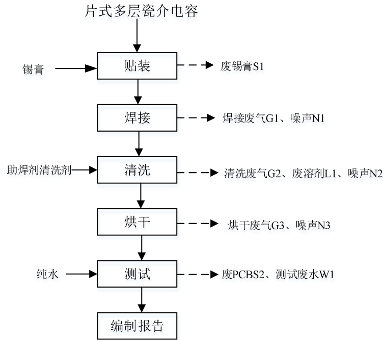
图 2-3 项目生产工艺流程图
