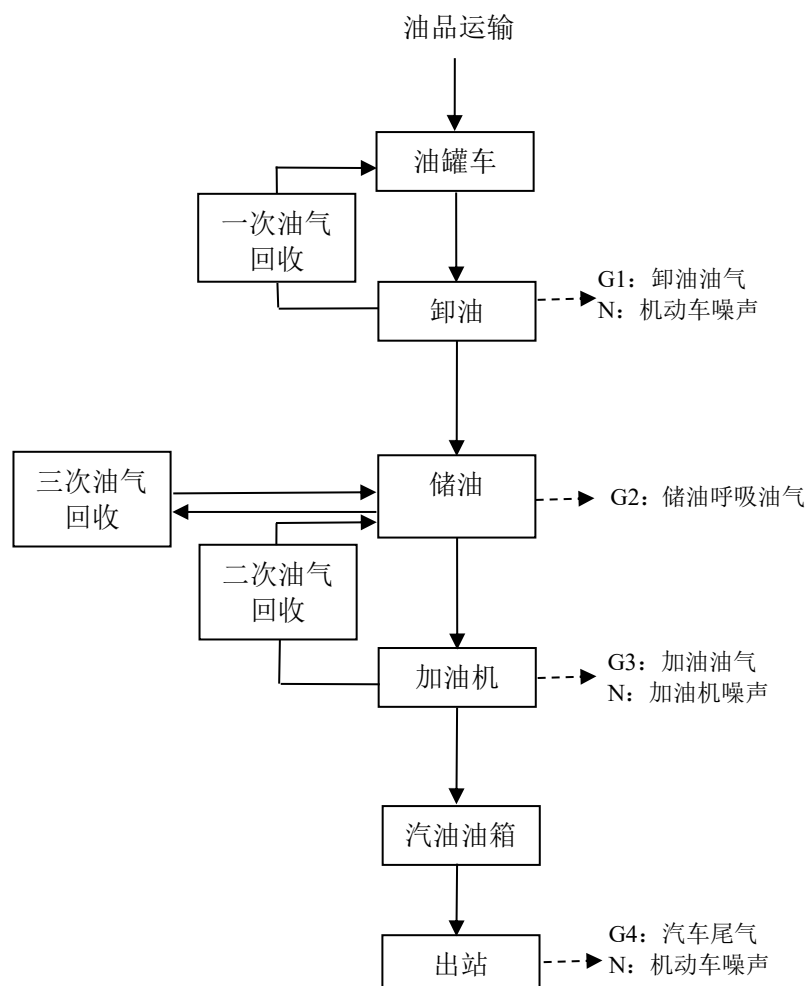
图2-3 加油站工艺流程及产污环节图（G-废气；W-废水；N-噪声） 工艺简述：
