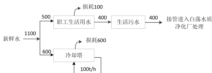
图 4-2 本项目水平衡图 (t/a)
