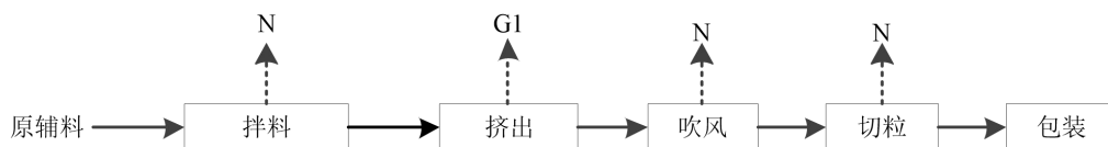
图 2-2 原有项目生产工艺流程图
