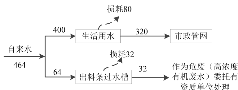
图 2-3 现有项目水平衡图
