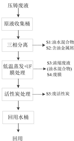
图 2-3 压铸废液处理工艺流程图
