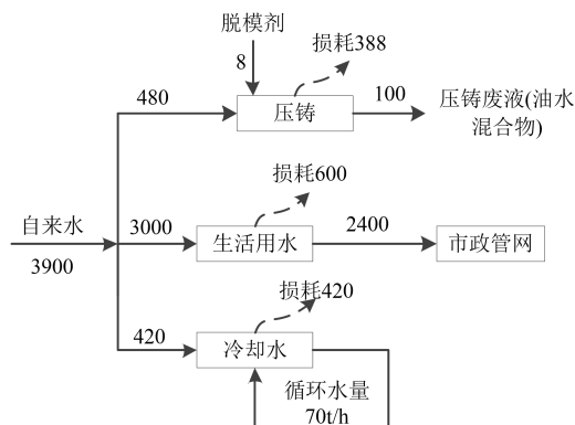
图 2-7 现有项目水平衡图
