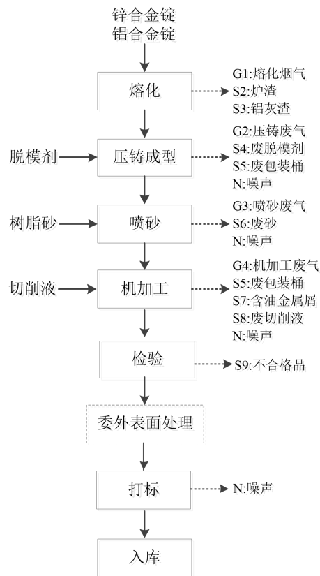
图 2-6 精密压铸件制造工艺流程
