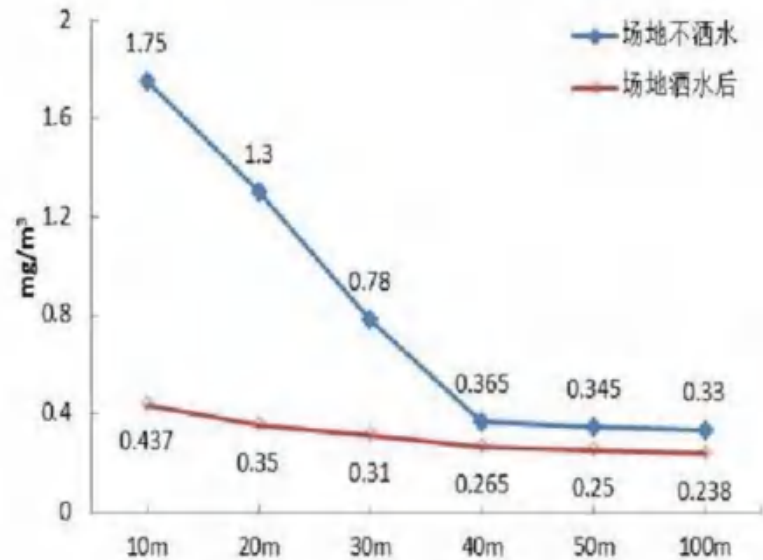
图 4-1 施工场界不同距离处 TSP 浓度变化
