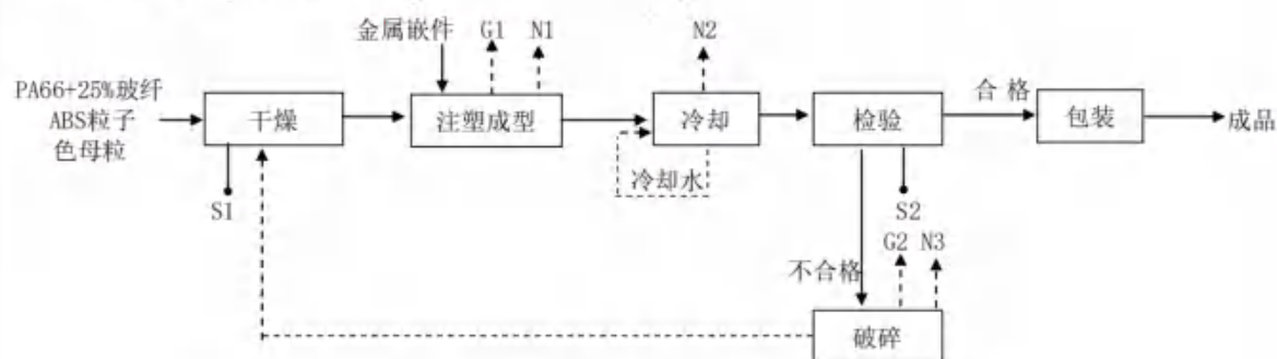
图 2-7 现有项目生产工艺流程图
