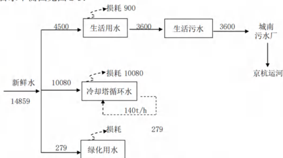
图 2-3 本项目水平衡图 (m³/a)
