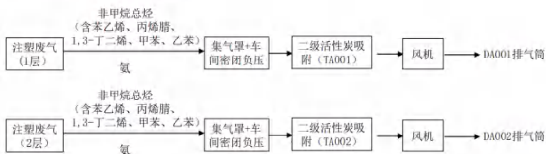
图 4-2 有组织废气收集处理工艺流程图
