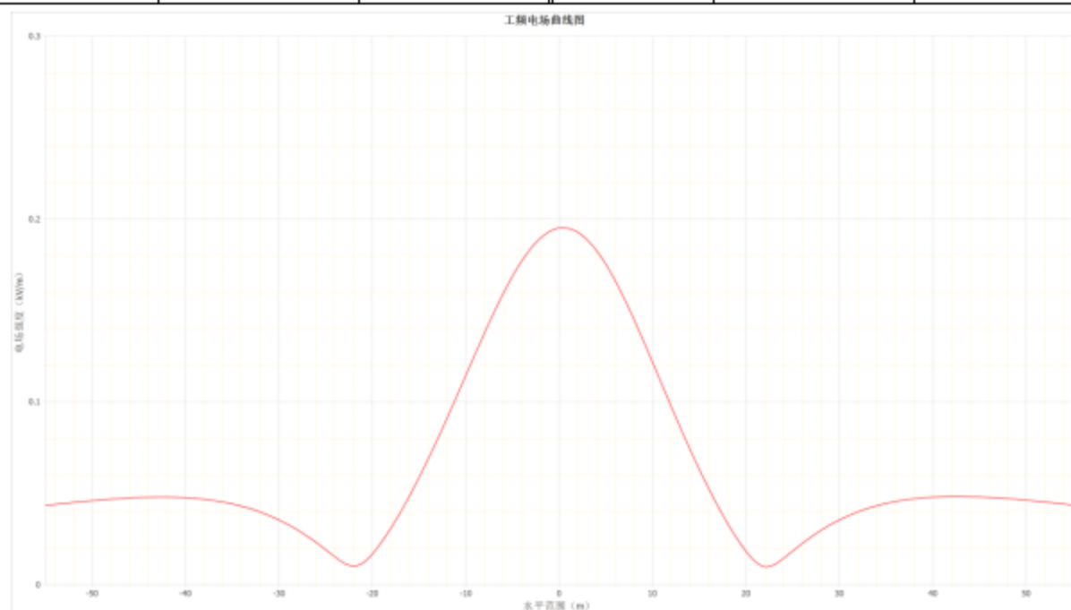
图 3-1 本项目架空线路下工频电场随距离变化趋势图
