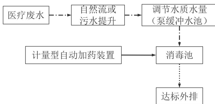
图 4-1 CLW-SD 型消毒设备污水处理流程图
