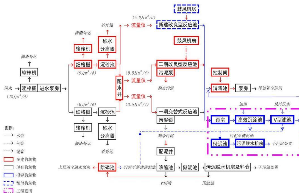
图 4-2 福星污水处理厂流程图
