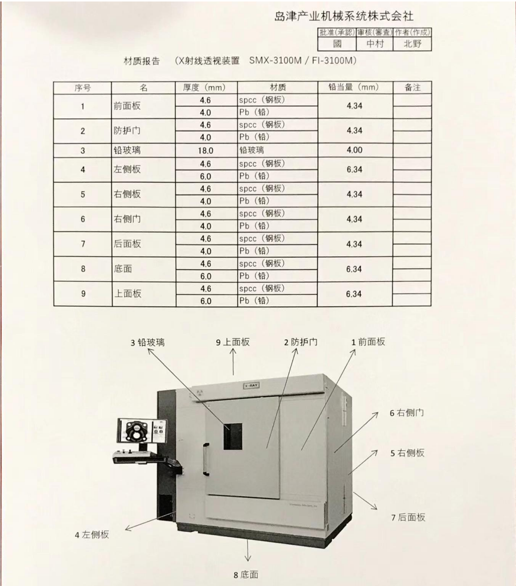
工业用 X 射线装置具体屏蔽措施见表 10-1。
