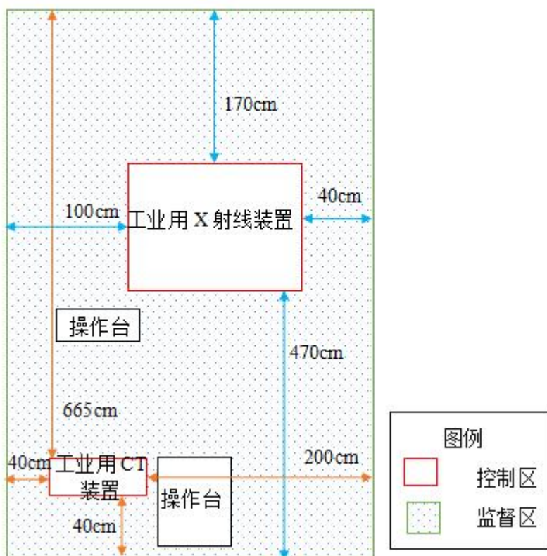
图 11-1 本项目工作场所辐射分区划分示意图
