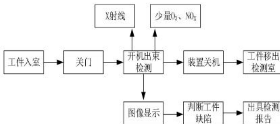
图 9-6 微焦点 X 射线透视检查装置工作流程及产污环节
