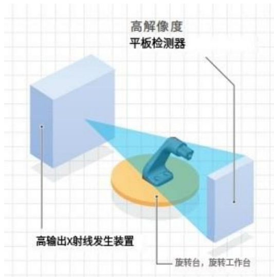
图 9-5 本项目工业 CT 扫描结构图
