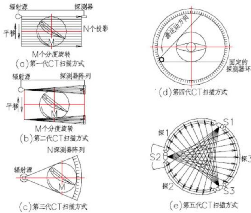
图 9-4 工业 CT 扫描结构
