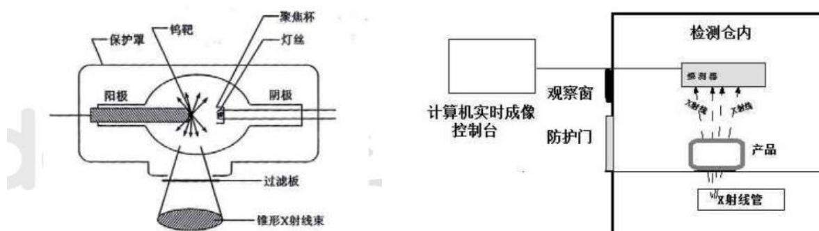
X 射线管线及 X 射线产生的示意图
