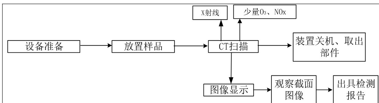
图 9-7 台式 X 射线 CT 系统工作流程及产污环节
