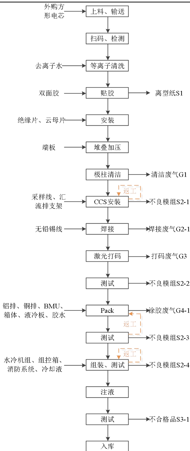
图 2-2 工商储（1F）生产工艺流程图
