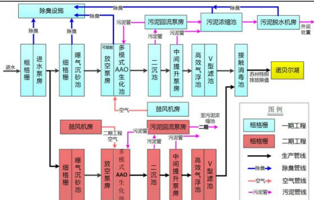
图 4-1 科技城水质净化厂处理工艺流程图
