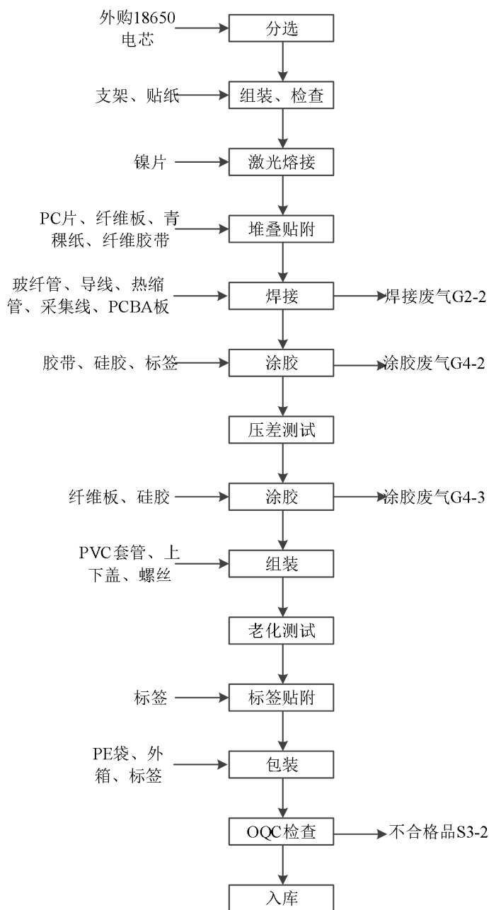
图 2-3 家储（2F）生产工艺流程图
