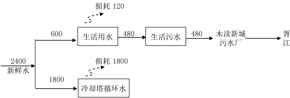
图 2-1 本项目水平衡图 (m³/a)
