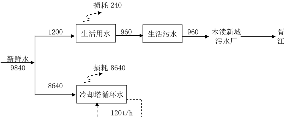
图 2-2 扩建后全厂水平衡图 (m³/a)
