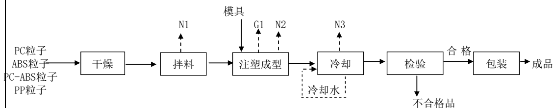
图 2-4 现有项目生产工艺流程图
