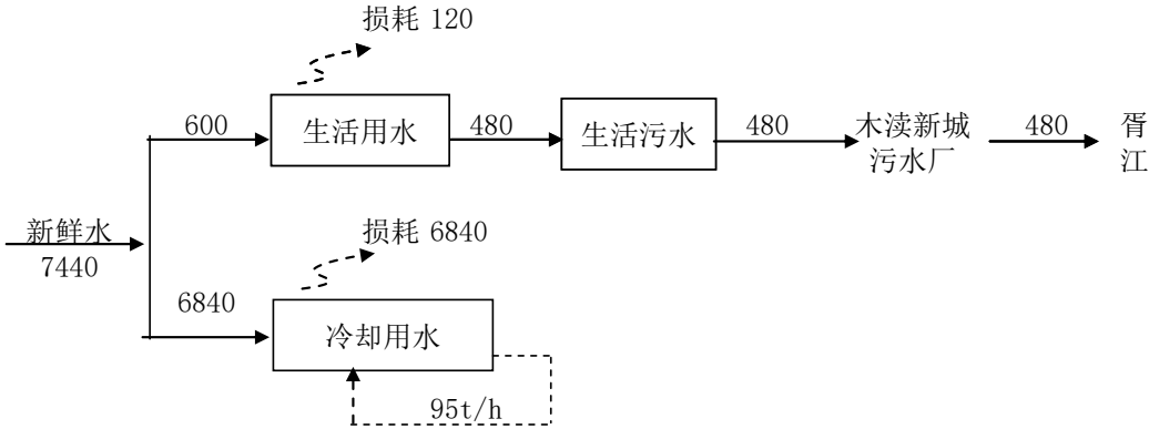
图 2-5 现有项目水平衡图 (m³/a)
