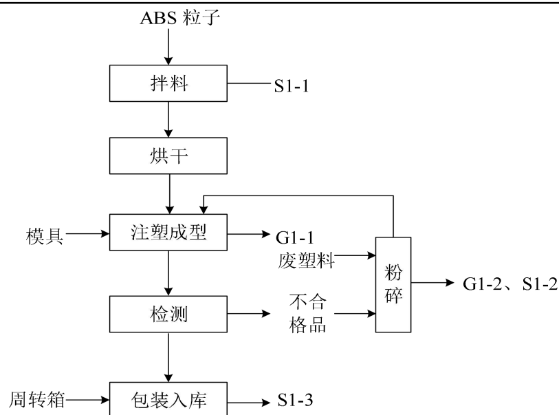
图 2-3 现有塑料制品生产工艺流程图
