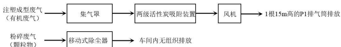
图 2-4 现有项目废气处理工艺流程图
