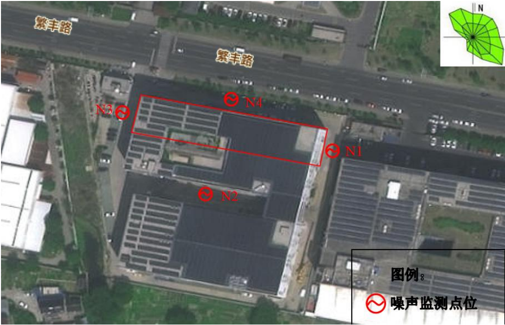
图 3-2 声环境现状监测图 表 3-6 声环境现状监测结果一览表
