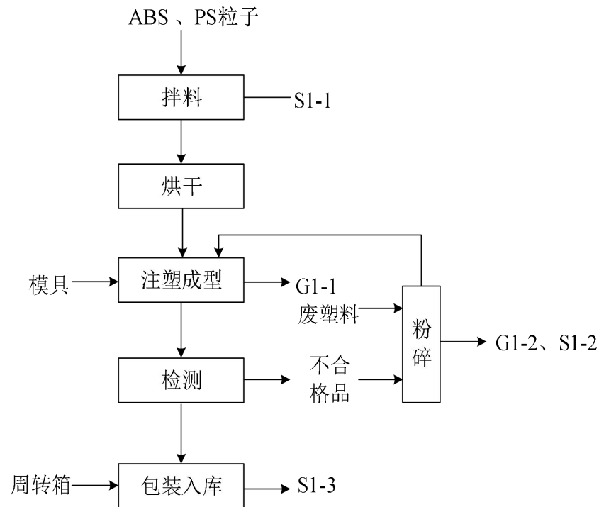
图 2-2 注塑件生产工艺流程
