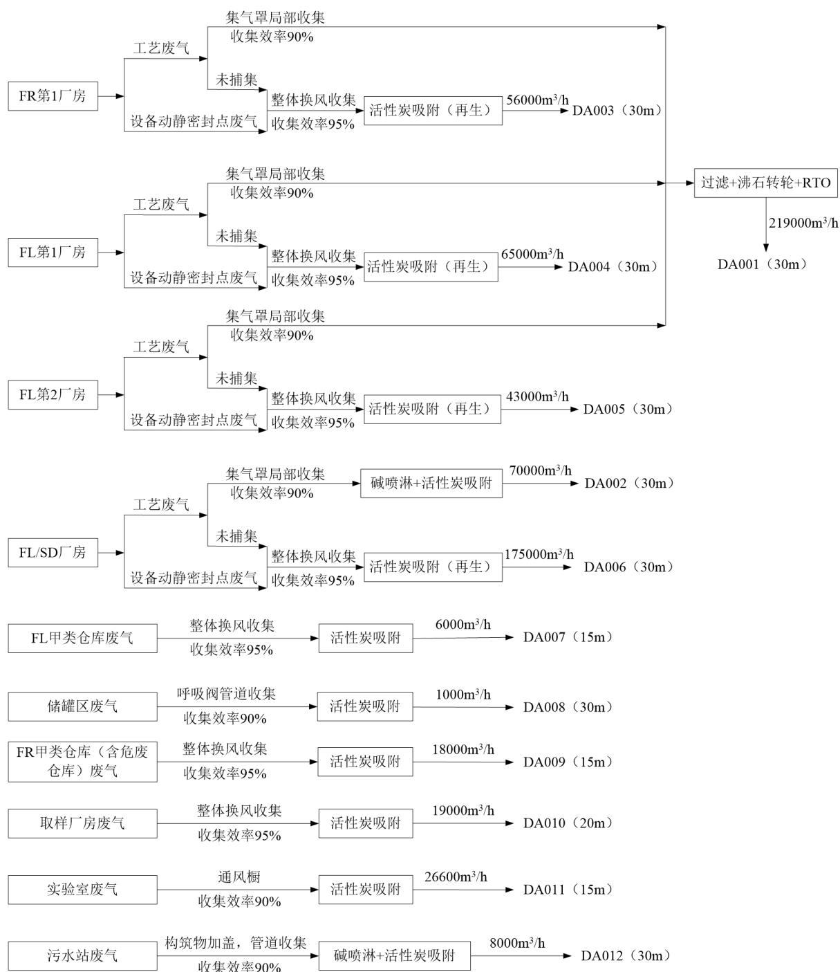
图 6.1.1.1-1 废气收集及处理流向图
