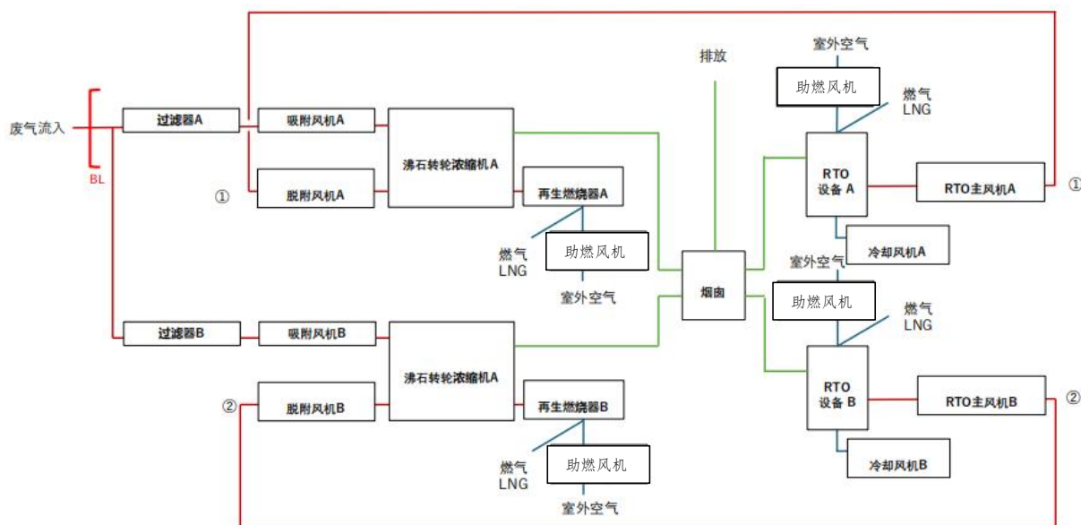
图 6.1.1.2-1: “过滤+沸石转轮+RTO”废气治理工艺流程简图
