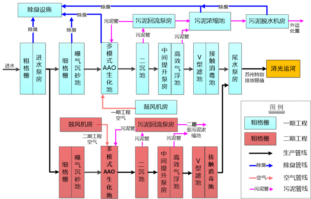
图 4-3 科技城水质净化厂污水处理流程图
