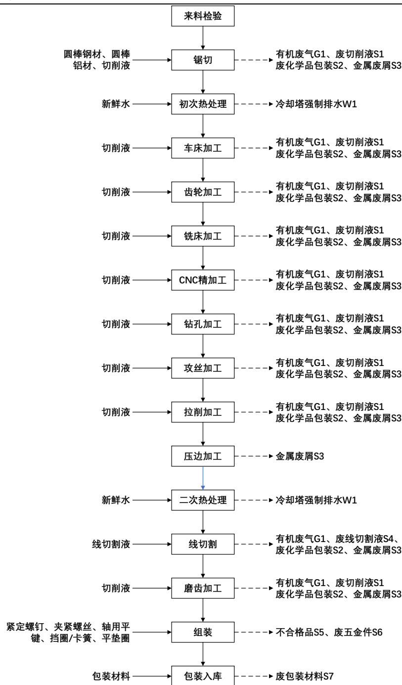
图 2-3 传动设备部件/产品工艺流程及产排污环节图
