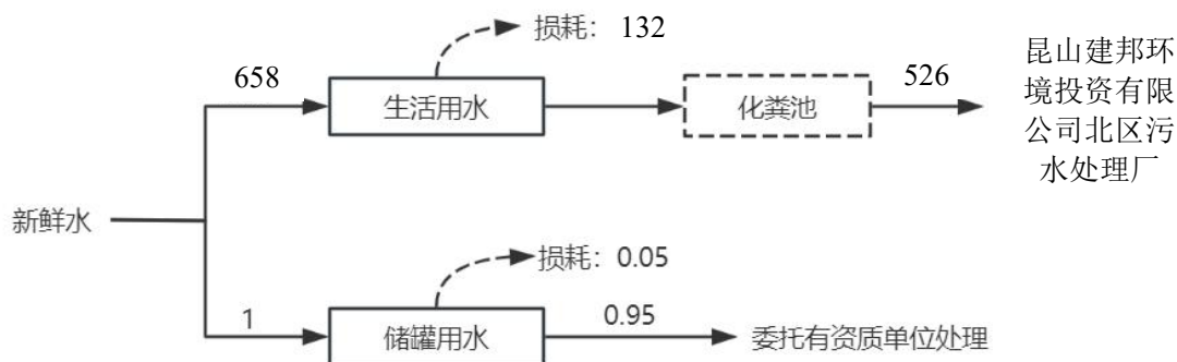
图 2-9 现有项目水平衡图 (单位: t/a)
