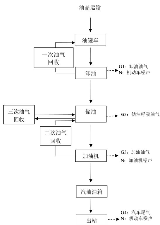
图 2-3 加油站工艺流程及产污环节图（G-废气；W-废水；N-噪声）
