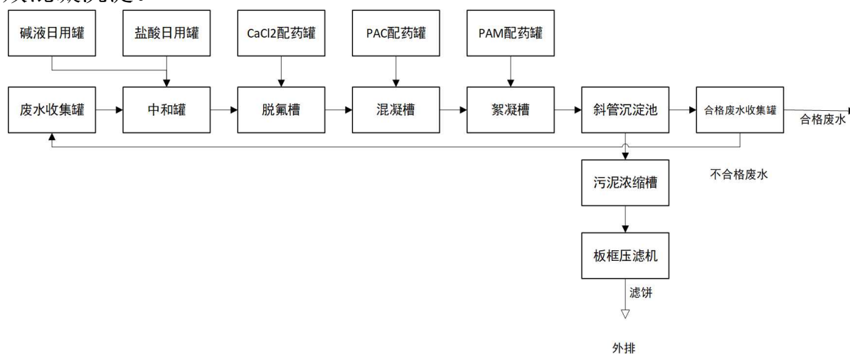
图6.2.2-1 含氟废水处理系统工艺流程示意图
