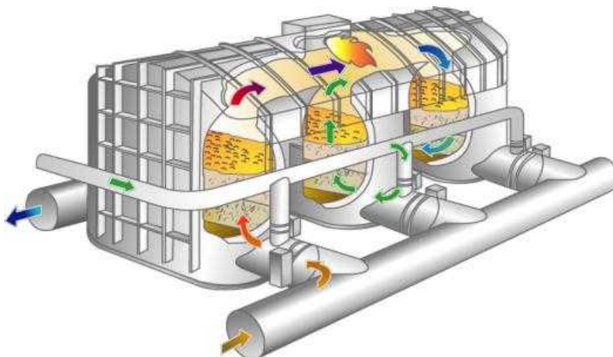
图 6.2.1-3 RTO 装置结构示意图
