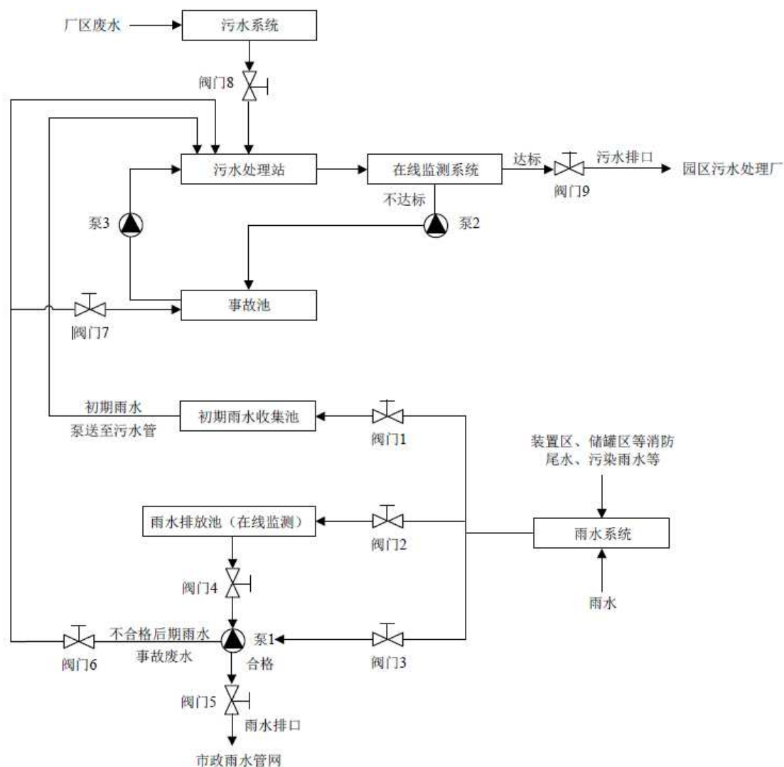
图 6.6.1-1 事故废水厂内管控示意图
