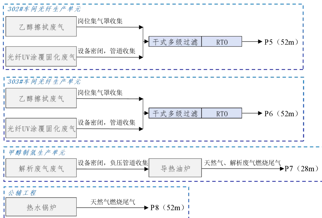
图 6.2.1-1 本项目涉及有组织废气收集及处理示意图
