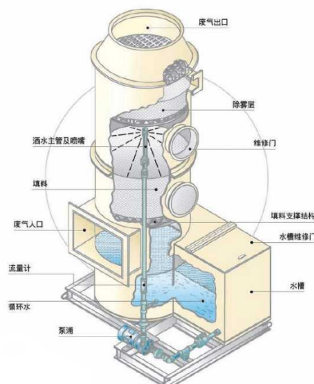
图 6.2.1-2 喷淋塔结构示意图
