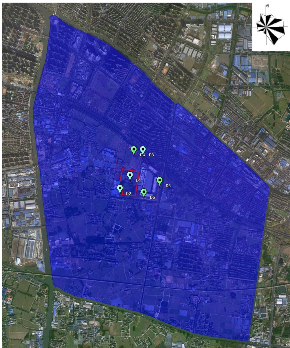
图 4.3.4-1 地下水监测点位图
