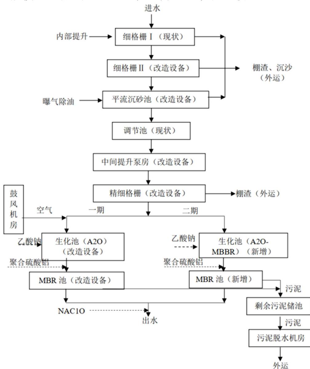
图 6.2.3-3 金港污水处理厂一期二期污水处理工艺流程图
