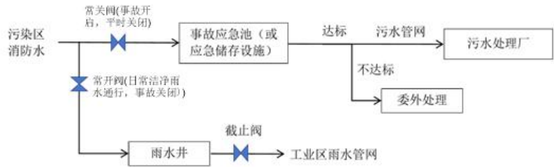
图 4-3 事故废水控制、封堵系统示意图
